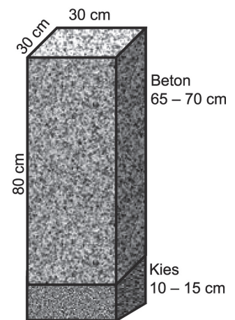
FUNDAMENT
